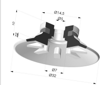
Ventosa plana Série 90 Ø 31,8 mm Referência do produto: 90 30-- A
