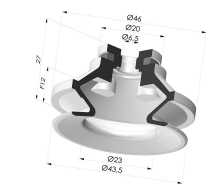
Ventosa 1.5 Fuelles Serie 91 Ø 40MM Referencia del producto: 91 40-- A
