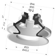
Ventosa 1.5 Fuelles Serie 91 Ø 40MM
