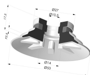
Ventosa Plana Serie 90 Ø 53MM Referencia del producto: 90 50-- A
