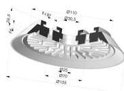
Ventosa Plana Serie 90 Ø 150MM Referencia del producto: 90 150-- A
