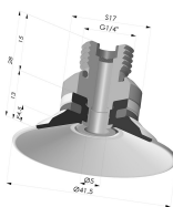
Ventosa Plana Serie 9 Ø 41.5MM
