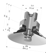
Ventosa Plana Serie 9 Ø 41.5MM
