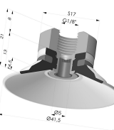
Ventosa Plana Serie 9 Ø 41.5MM
