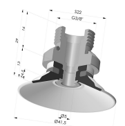
Ventosa Plana Serie 9 Ø 41.5MM
