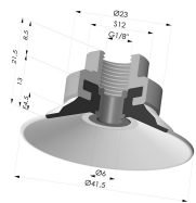
Ventosa Plana Serie 9 Ø 41.5MM
