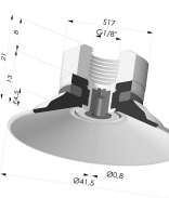
Ventosa Plana Serie 9 Ø 41.5MM
