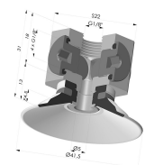
Ventosa Plana Serie 9 Ø 41.5MM
