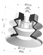
Ventosa 2.5 Fuelles Serie 96C Ø 25MM
