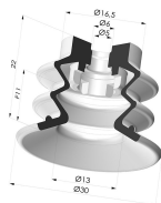
Ventosa 2.5 Fuelles Serie 96B Ø 30MM
