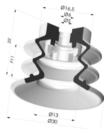
Ventosa 2.5 Fuelles Serie 96C Ø 30MM
