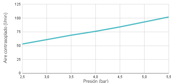
AIRE CONTRASOPLO EN FUNCIÓN DE LA PRESIÓN
