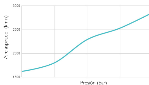
AIRE ASPIRADO EN FUNCIÓN DE LA PRESIÓN *
